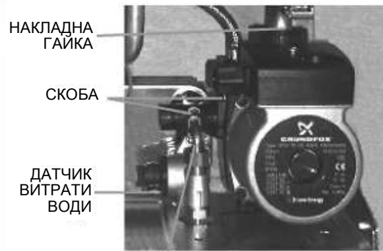
З'ЄДНУВАЛЬНИЙ КЛАПАН ПІДЖИВЛЮЮЧОГО ВЕНТИЛЯ
